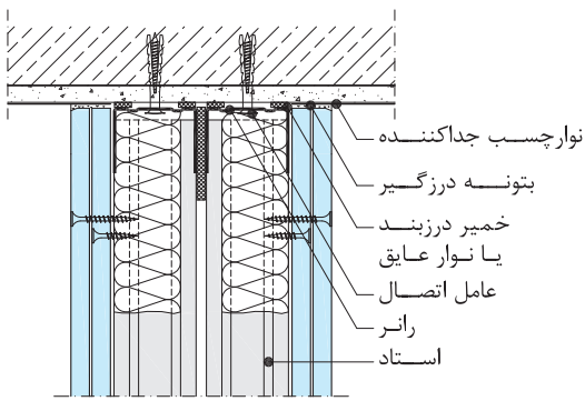
اتصال به سقف
