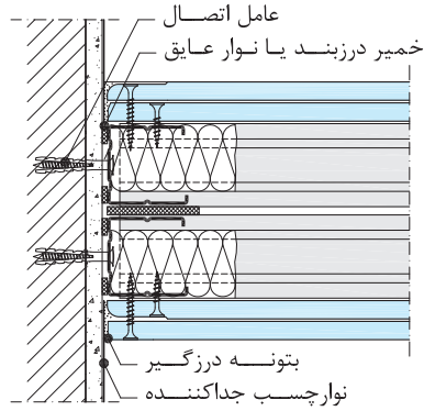
اتصال به دیوار بنایی جانبی
