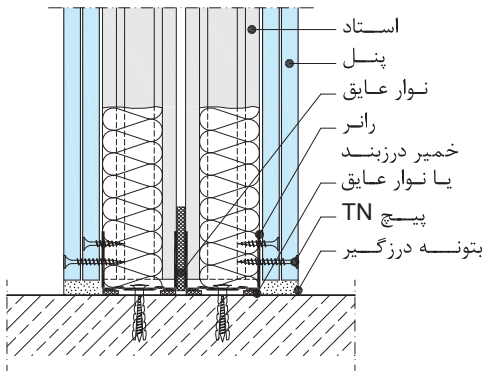
اتصال به کف
