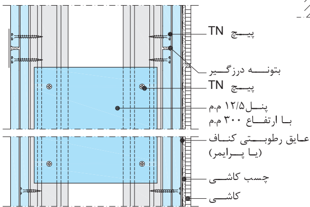
درز افقی و نحوه اتصال استاداها
