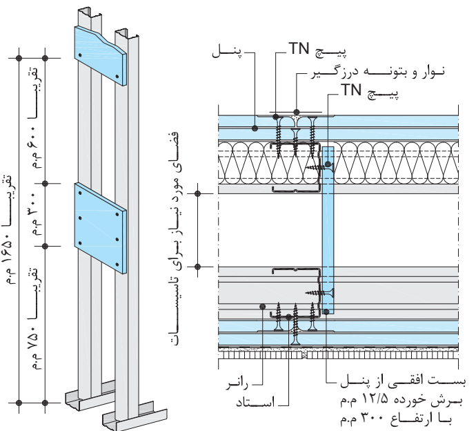
نحوه اتصال استاداها
