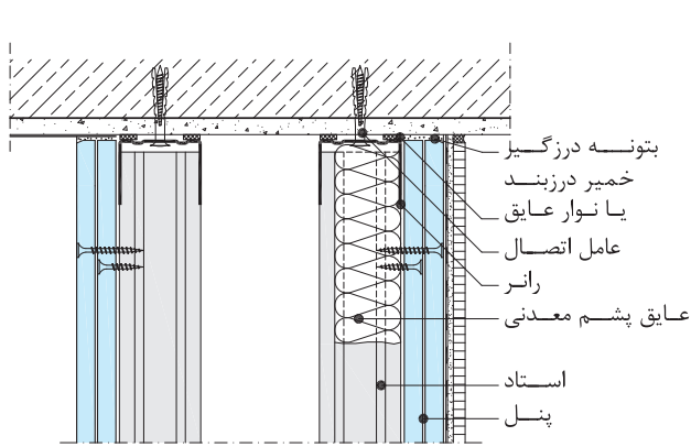
اتصال به سقف
