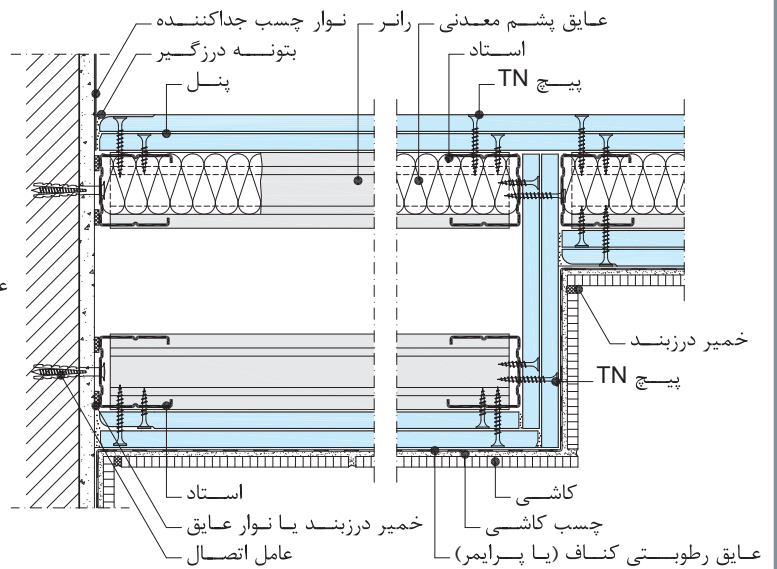
اتصال به دیوار بنیایی جانبی و تغییر ضخامت دیوار
