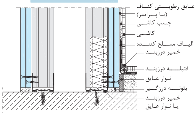
اتصال به کف (دیوار دو لایه با عایق کم ضخامت)
