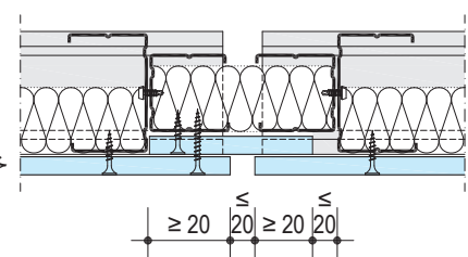
درز انقطاع با اتصال کشویی لغزان
