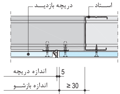
جزئیات نصب دریچه بازدید
