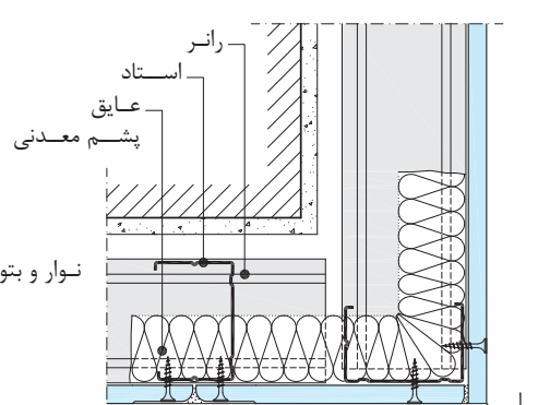
سازه (یا نوار) محافظ گوشه
