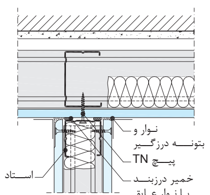
اتصال دیوار جداکننده به دیوار پوششی
