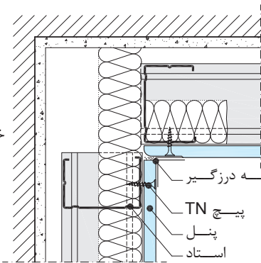
اتصال گوشه داخلی و خارجی
