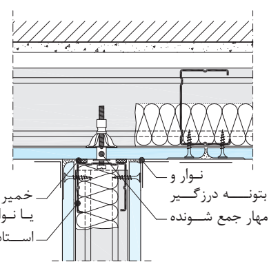
اتصال دیوار جداکننده به دیوار پوششی
