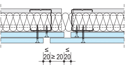
اتصال دیوار جداکننده به دیوار پوششی
