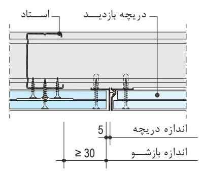
جزئیات نصب دریچه بازدید
