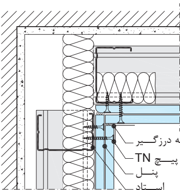
اتصال گوشه داخلی و خارجی
