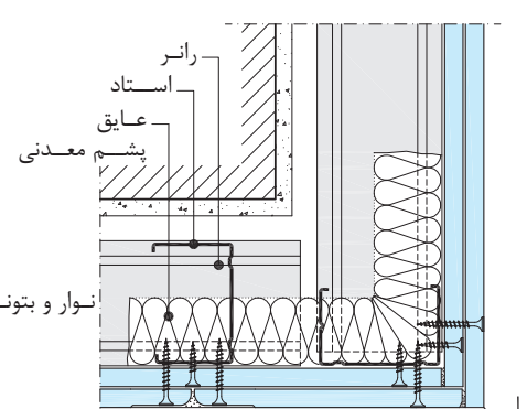
سازه (یا نوار) محافظ گوشه
