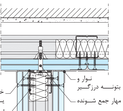
اتصال گوشه داخلی و خارجی
