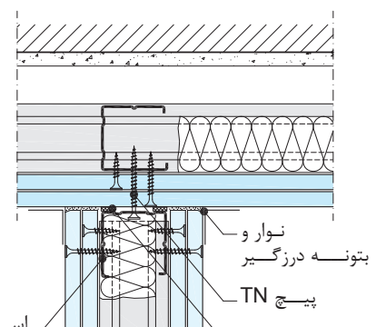
اتصال دیوار جداکننده به دیوار پوششی
