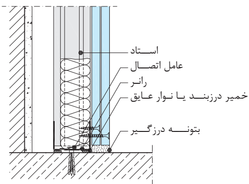
اتصال به کف
