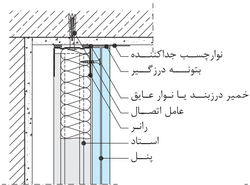
اتصال به سقف
