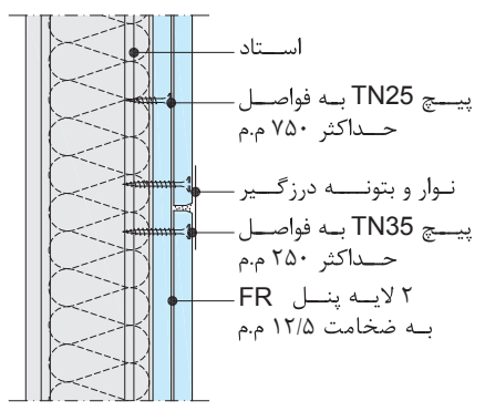
درز افقی
