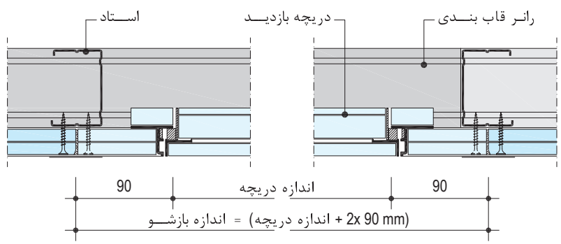
جزئیات نصب دریچه بازدید
