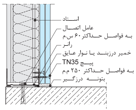
اتصال به کف
