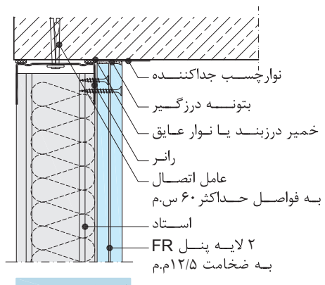
اتصال به سقف
