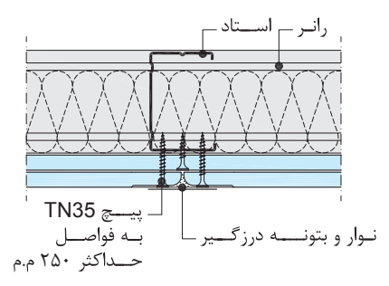
درز قائم
