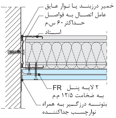
اتصال به دیوار بنایی جانبی
