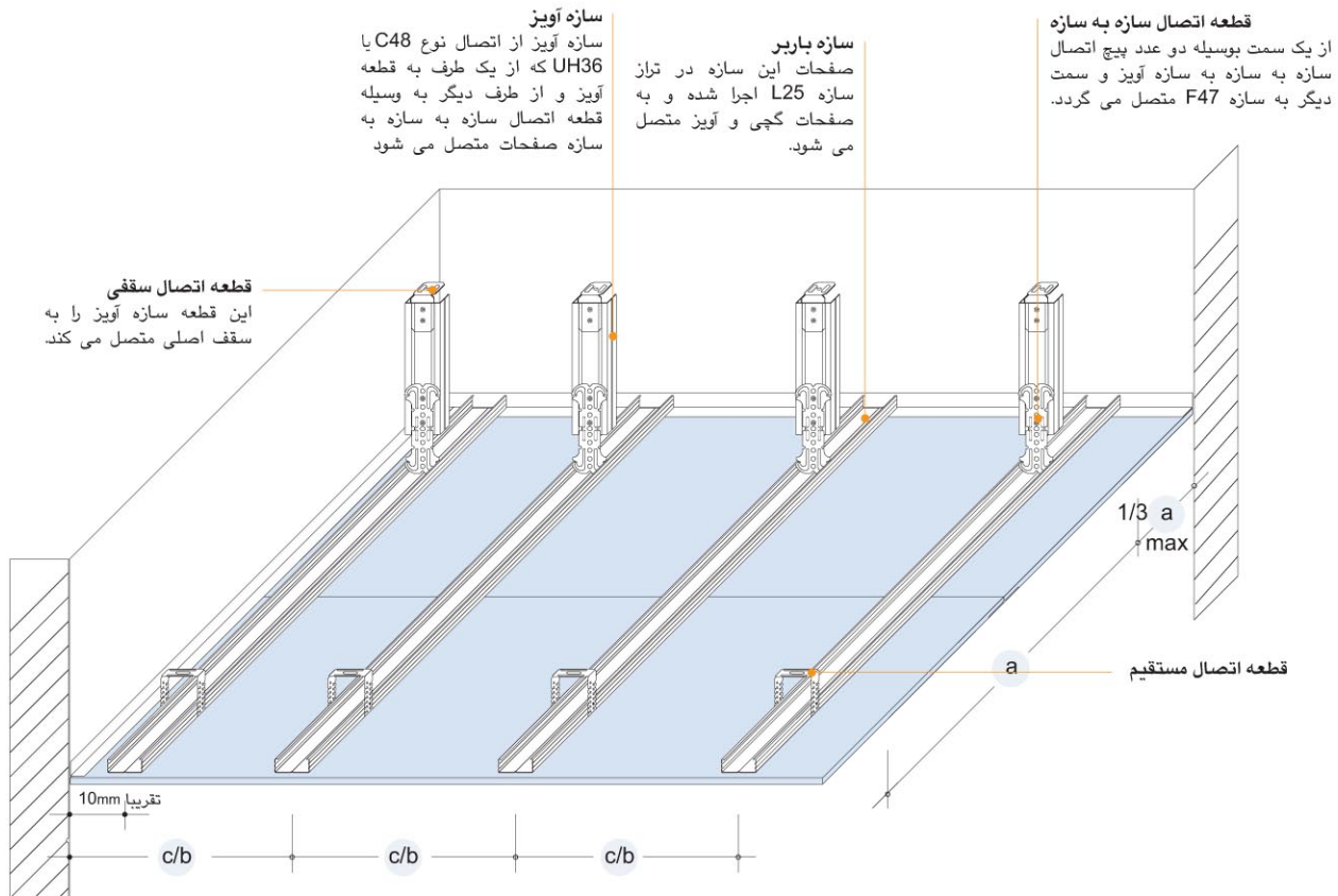
فاصله اجزاء سازه با توجه به رده وزنی در سقفهای D112I(B)
